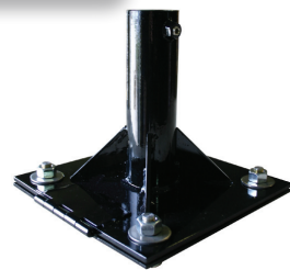
Fig. 610 Hinged Base 610B--0200 AB
